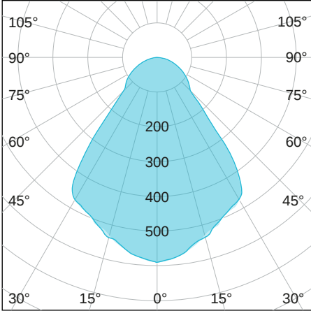
LICHTVERTEILUNGSKURVE
