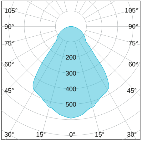
LICHTVERTEILUNGSKURVE
