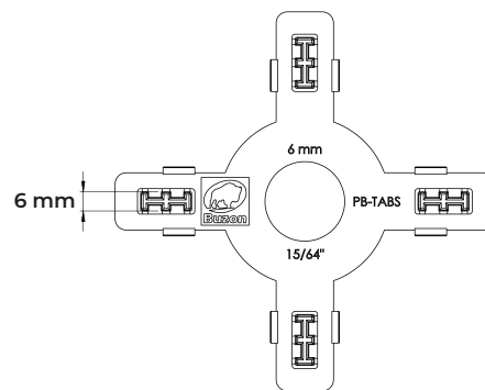
PB-TABS
