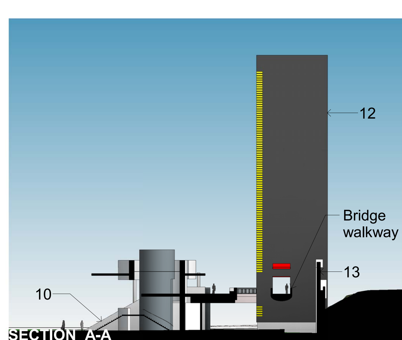
SECTION A-A
