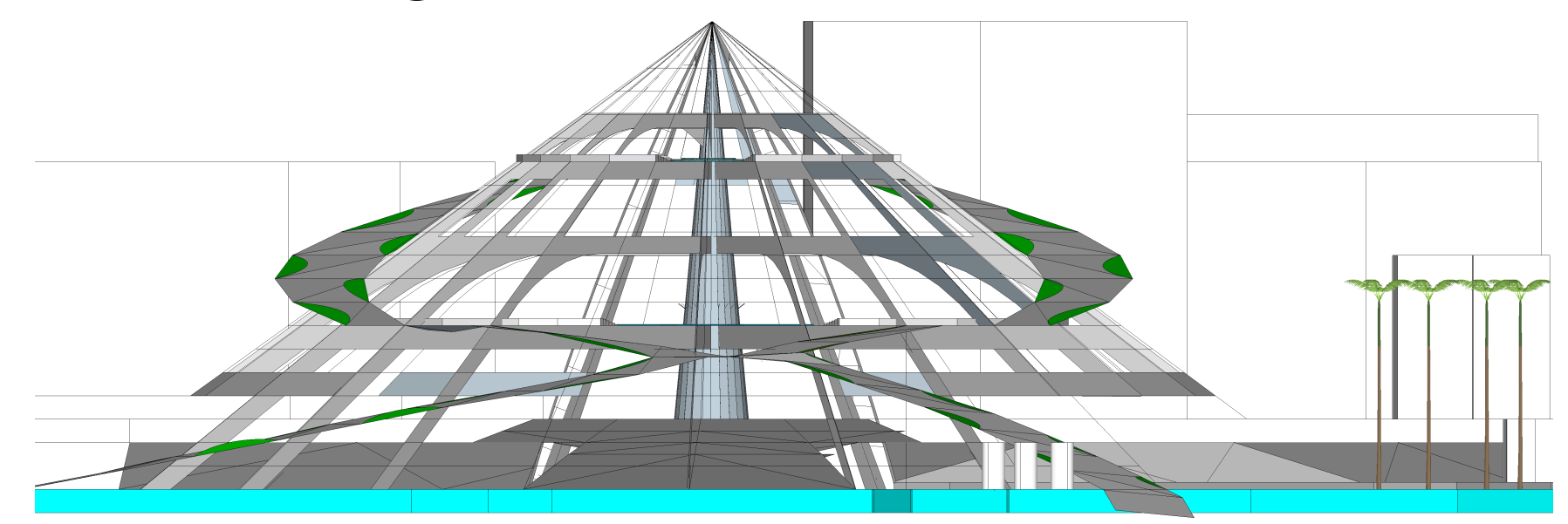
ELEVATION FROM N. AUTOMN ST.
