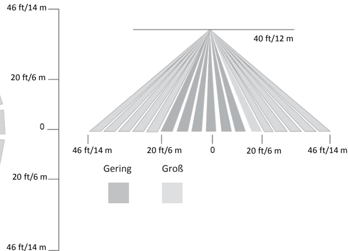
Seitenansicht
