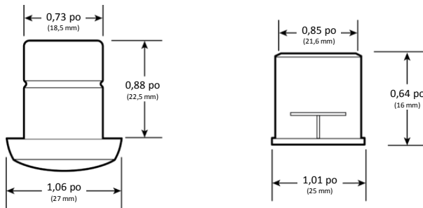
Micro-capteur (SU-5E)
