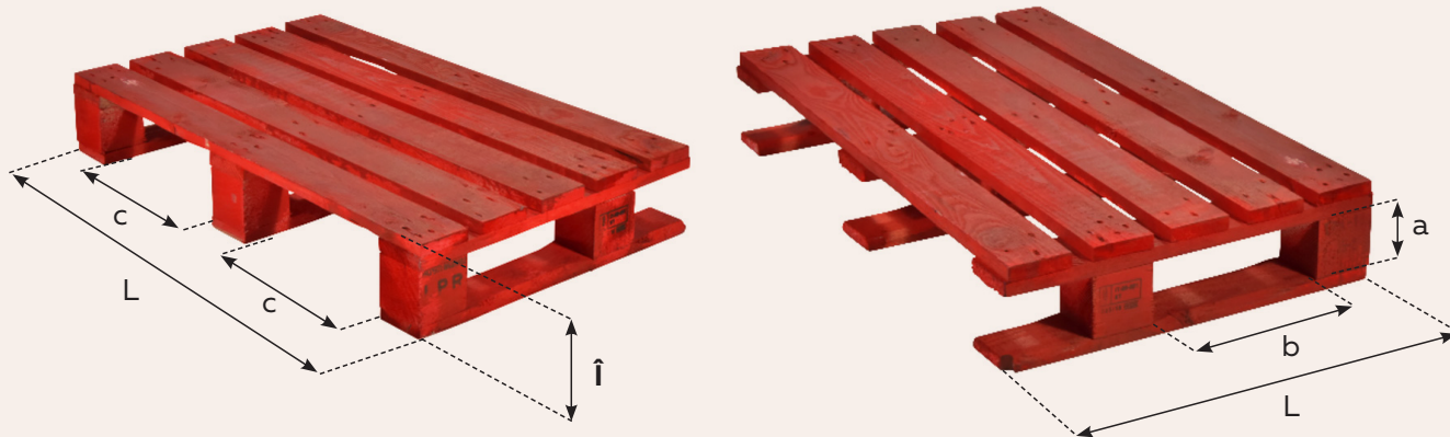
DP610 - Dimensiuni nominale și toleranța paleților (mm)
