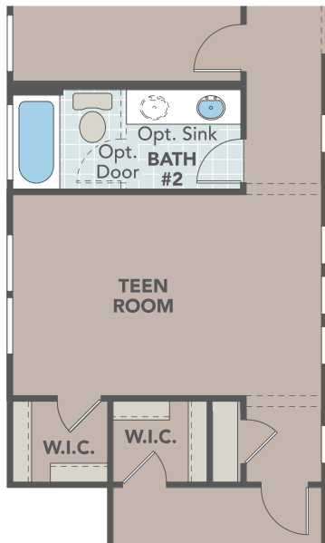
Optional Teen Room ILO Bedroom #3
