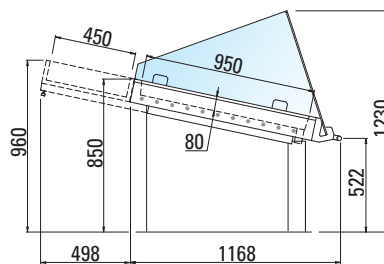
Letto di ghiaccio con serpentina Ice bed with cooling coil
