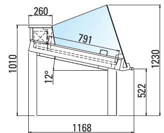
con evaporatore with evaporator
