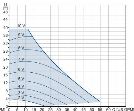
0-10 volts*
