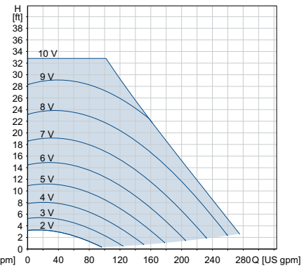
0-10 volts*
